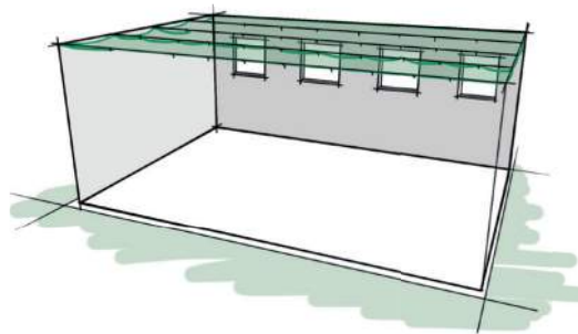
Beskyttelsesnett i taket av idrettshallen
