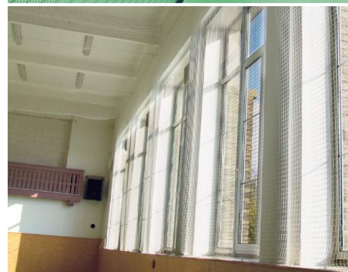
Egnet som skillenett i tennishaller, gymsaler og sportsbaner, backstop og beskyttelsesnett for ishockeystadioner over pleksiglasset. Materiale PA; maskestørrelse 40mm, nettykkelse 1,2 eller 2mm, farge: hvit, beige, svart
