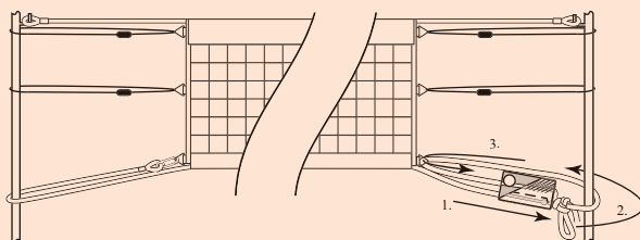
Teknikk for oppheng av volleyballnett (LIGA):
